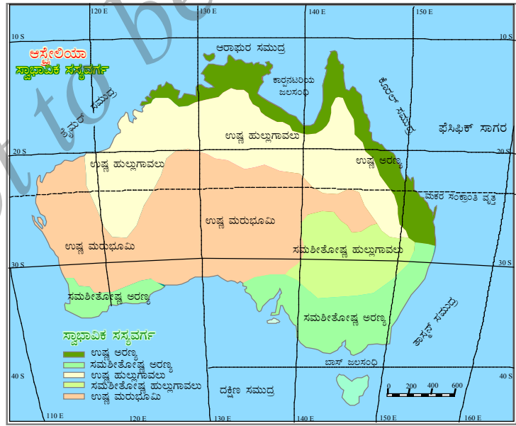
ಆಸ್ಟ್ರೇಲಿಯದ ಸ್ವಾಭಾವಿಕ ಸಸ್ಯವರ್ಗ
