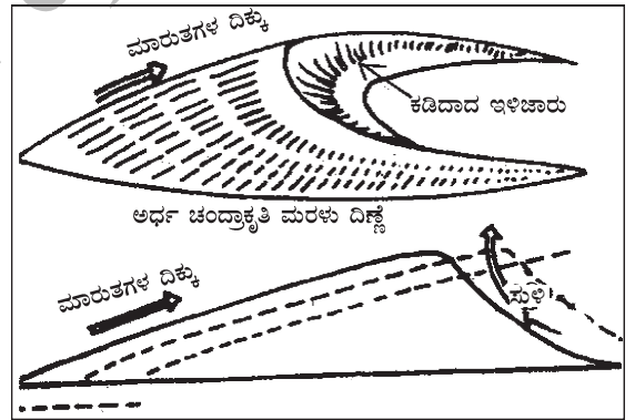
ಅರ್ಧಚಂದ್ರಾಕೃತಿಯ ಮರುಳುದಿಣ್ಣೆ
