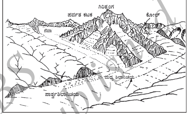
ಹಿಮನದಿ
