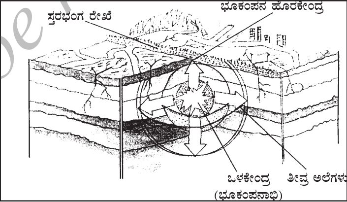
ಭೂಕಂಪದ ಕ್ರಿಯೆಗಳು
