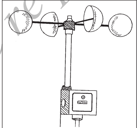
ಪವನ ವೇಗಮಾಪಕ
