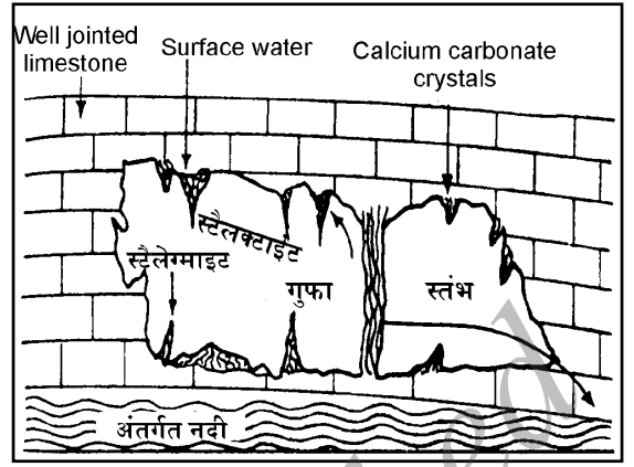
भूम्यांतर्गत पाणी
