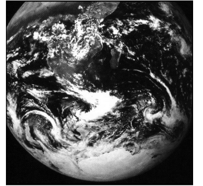
पृथ्वी
