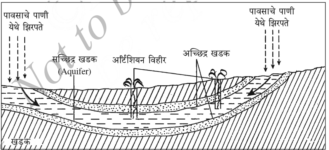
आर्टिशियन विहीर
