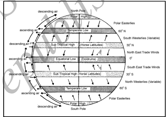
वाऱ्यांचे प्रकार
