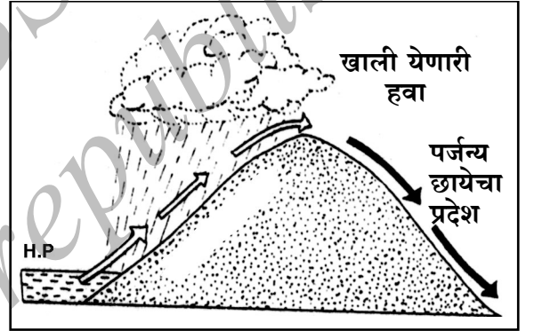
प्रतिरोध पर्जन्य
