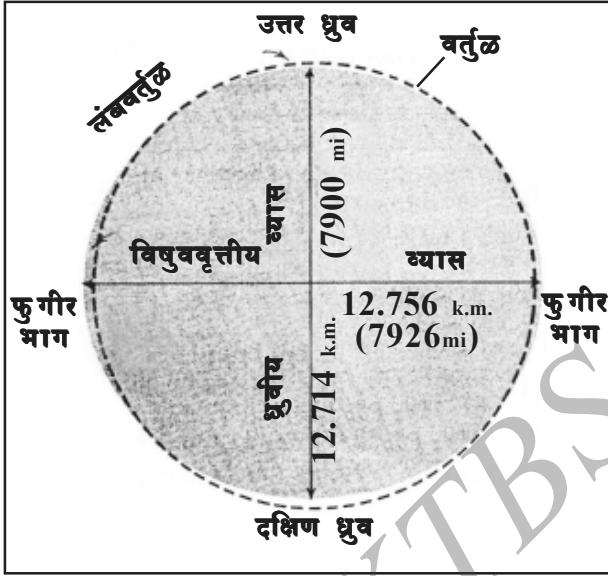
पृथ्वीचा आकार
