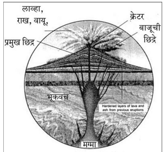
ज्वालामुखीची रचना
