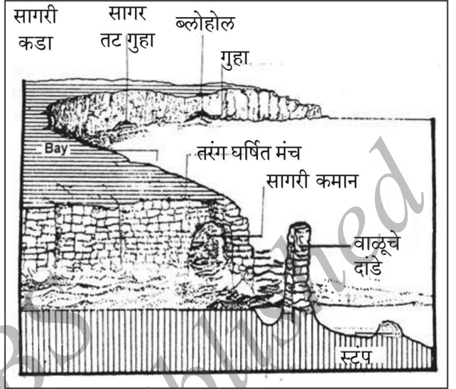
सागरी लाटा
