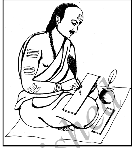
नाडोज पंप
