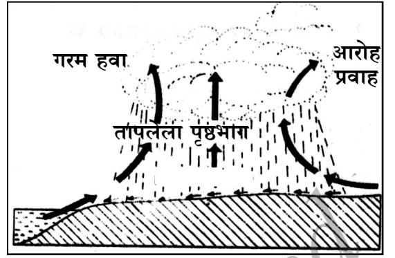
आरोह पाऊस
