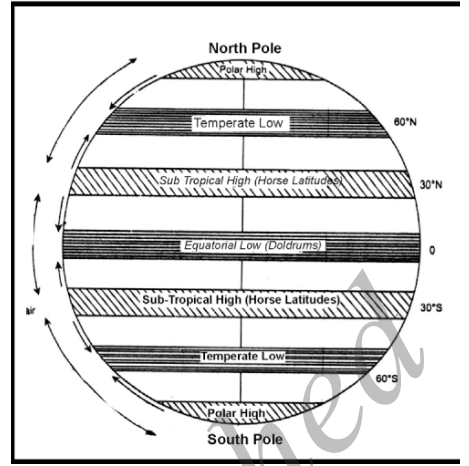
वायुदाबा पट्टे
