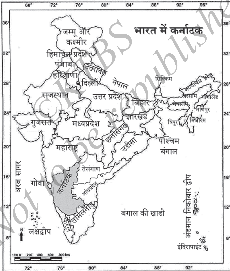
भारत में कर्नाटक का स्थानांकन
