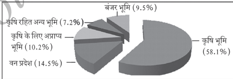
विविध भू-उपयोग के प्रतिशत भाग
